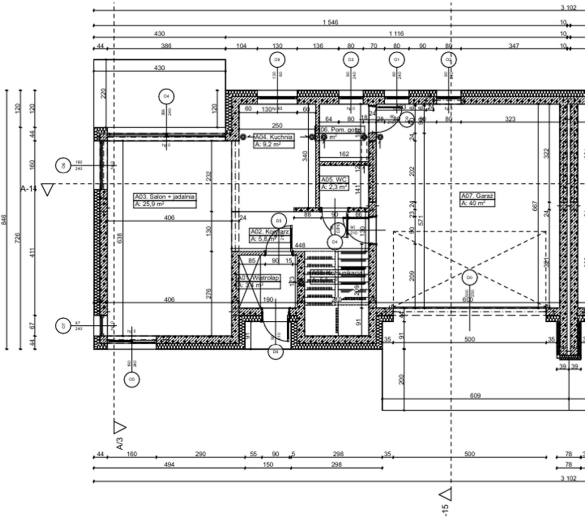
RZUT PARTERU
