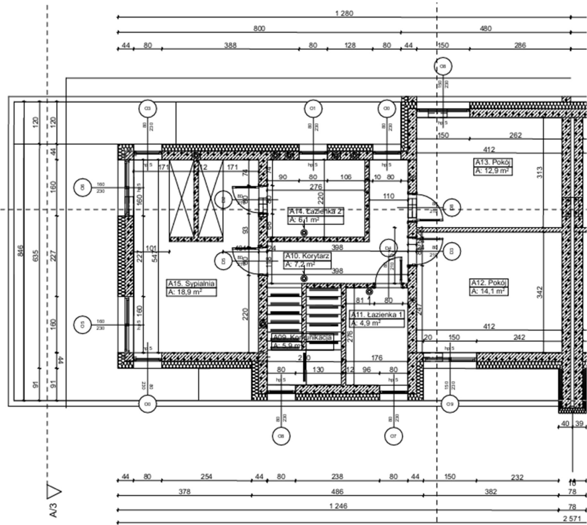
RZUT PIĘTRA
