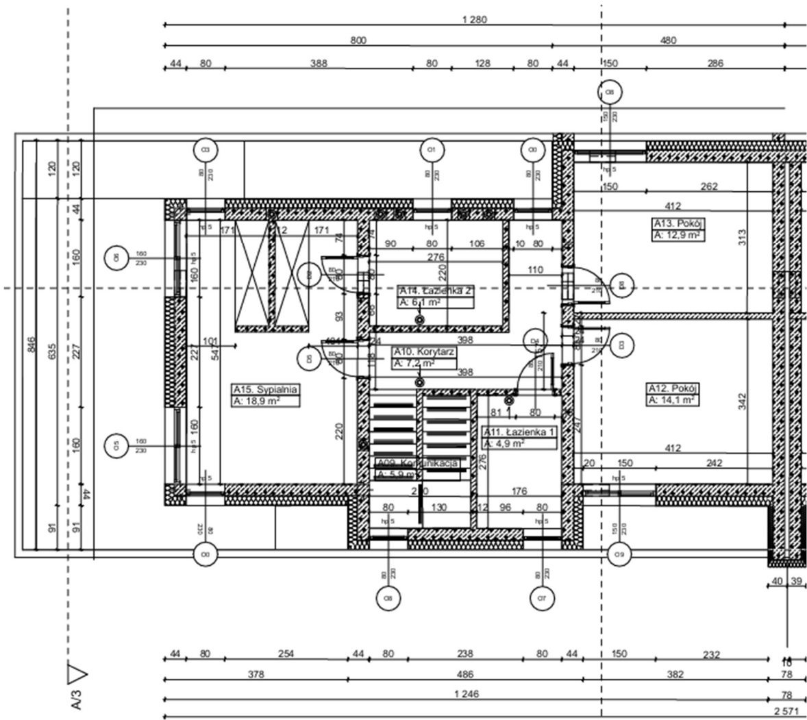
RZUT PIĘTRA
