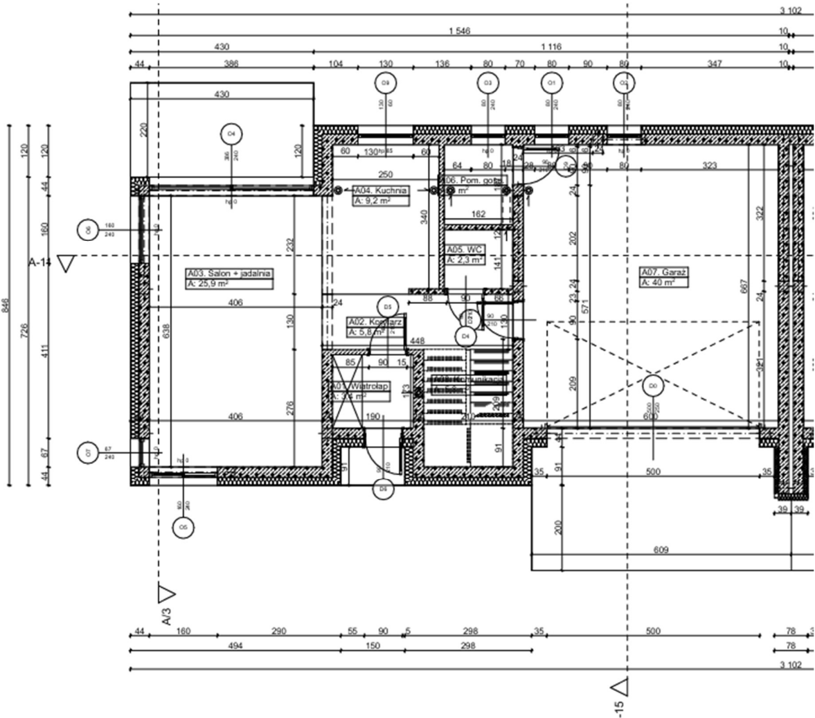
RZUT PARTERU
